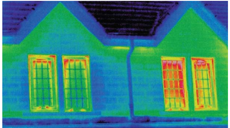
термална снимка: левите прозорци имат щори с BlackOut плат
