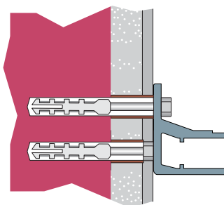
Монтаж в стена с изолация (трябва да се сложат втулки, за да не се смачка изолацията от планката)
