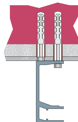
Монтаж в таван с изолация (трябва да се сложат втулки, за да не се смачка изолацията от планката)
