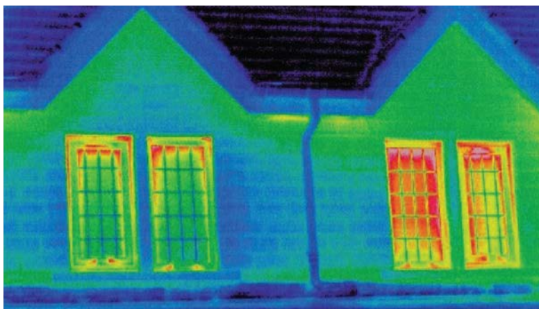
термална снимка: левите прозорци имат щори с BlackOut плат
